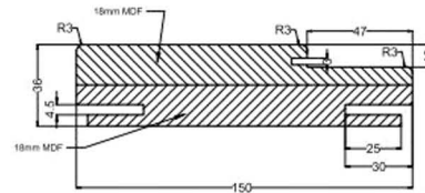
36x150x2100 BOMBELİ KASA (DÜZ ve 3D YÜZEY)
