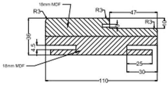
36x110x2100 BOMBELİ KASA (DÜZ ve 3D YÜZEY)
