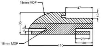
36x110x2100 BOMBELİ KASA (DÜZ ve 3D YÜZEY)
