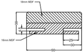
36x90x2100 BİRLEŞTİRME (DÜZ ve 3D YÜZEY)
