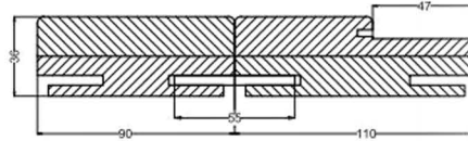
36x200x2100 BİRLEŞTİRME (DÜZ ve 3D YÜZEY)
