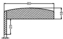
18x80x2200 BOMBELİ PERVAZ (DÜZ ve 3D YÜZEY)
