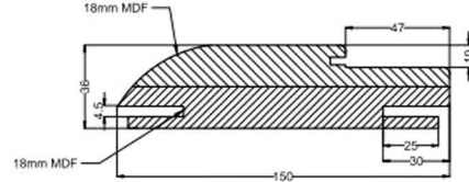
36x150x2100 BOMBELİ KASA (DÜZ ve 3D YÜZEY)
